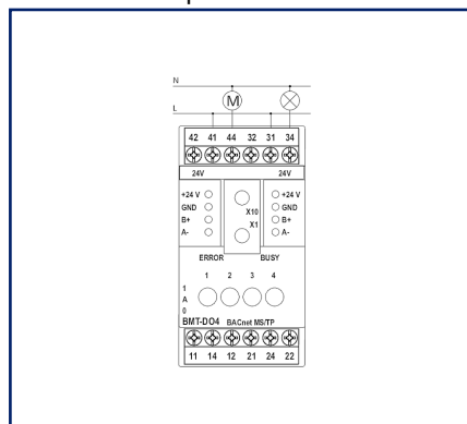
Anschlussbeispiel
