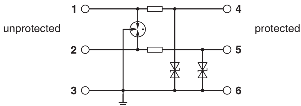
Diagrama eléctrico
