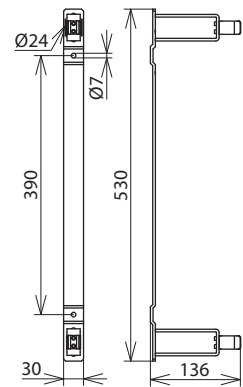
Maßbild HV P ST D24
