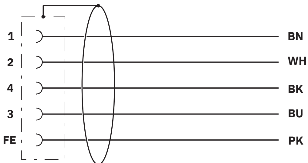
Diagrama eléctrico
