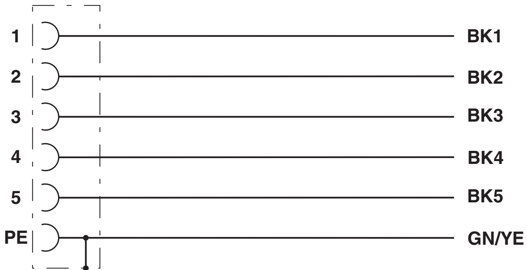
Schaltplan
