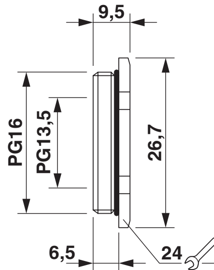
Maßzeichnung
