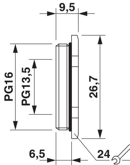
Esquema de dimensiones
