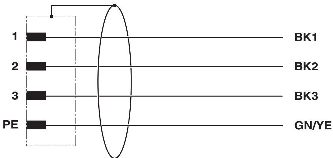
Diagrama eléctrico
