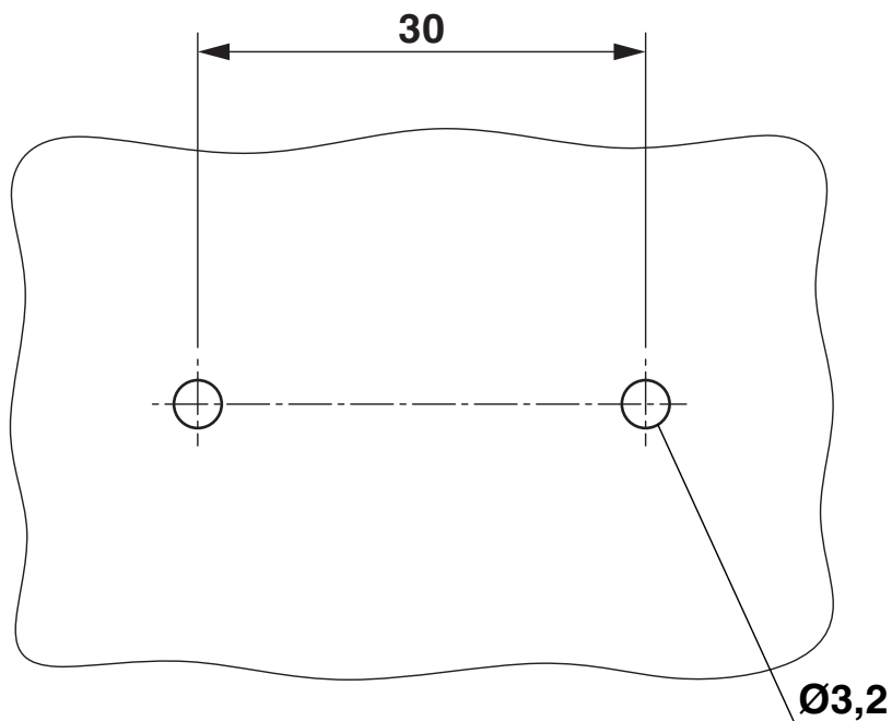
Dessin coté
