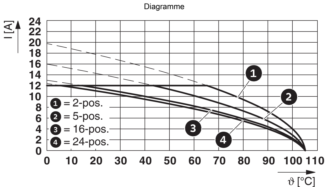
Type : ICV 2,5/...-G-5,08 avec MSTBVA 2,5/...-G-5,08
