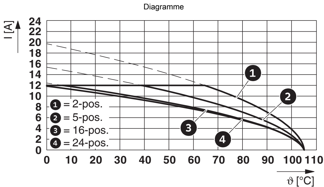
Type : IC 2,5/...-G-5,08 avec MSTBVA 2,5/...-G-5,08
