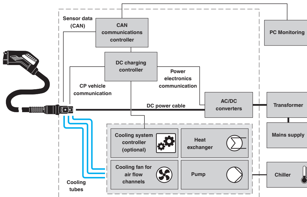
Schemazeichnung
