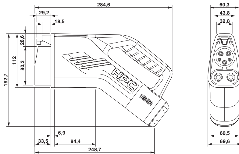
Dessin coté
