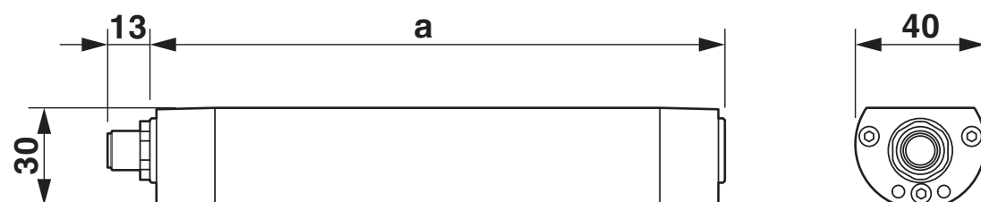
Esquema de dimensiones
