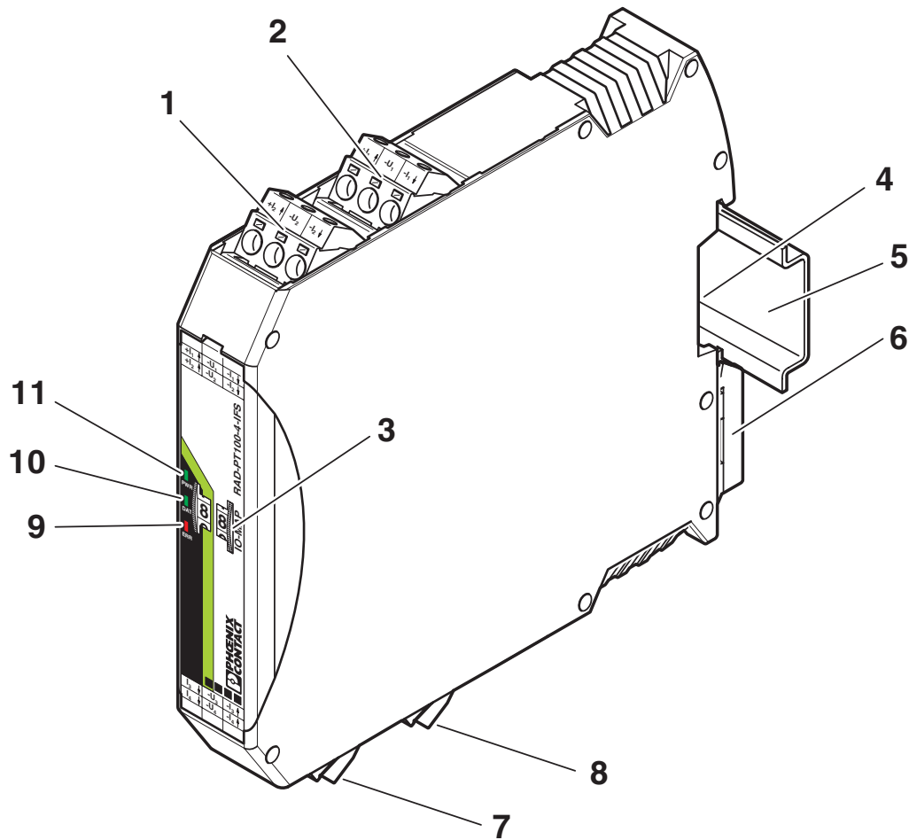
Plano esquemático
