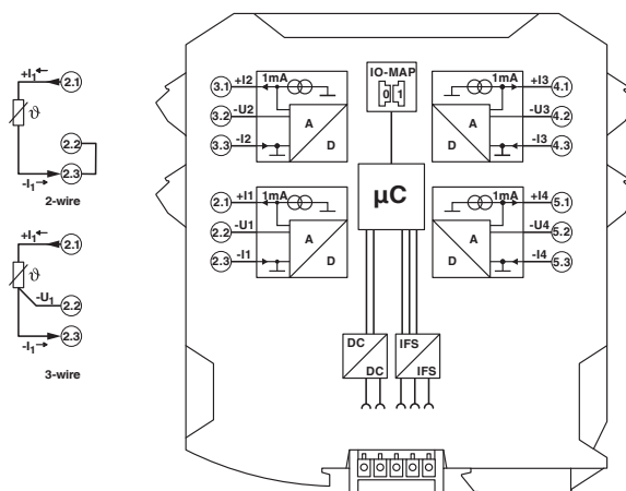
Diagrama eléctrico
