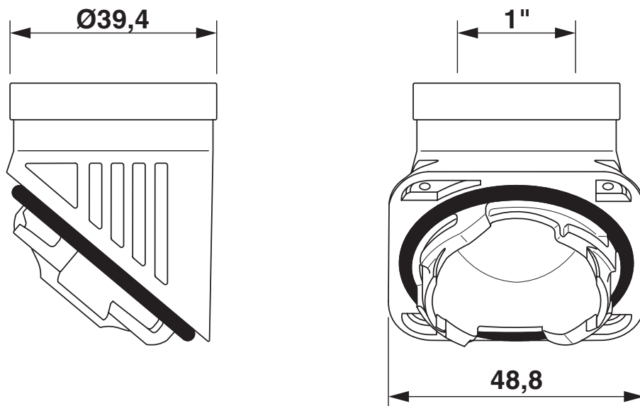
Maßzeichnung
