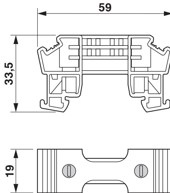
Dessin coté
