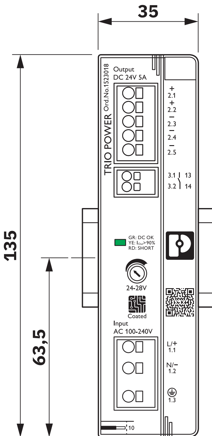
Esquema de dimensiones
