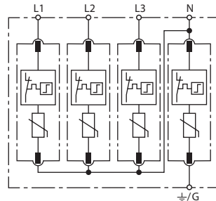
Prinzipschaltbild DG MU 3PY 208 4W+G
