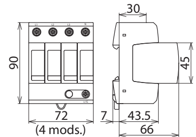
Maßbild DG MU 3PY 208 4W+G
