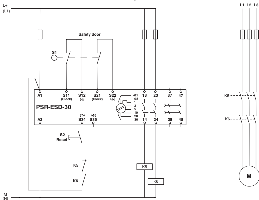
Zweikanalige Schutztürüberwachung
