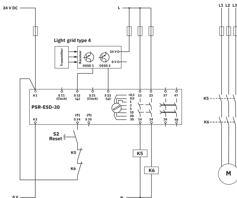
Schaltplan
