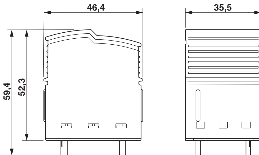
Dessin coté
