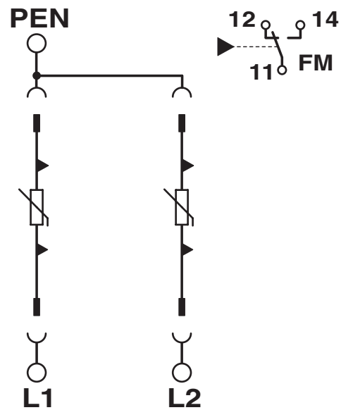
Diagrama eléctrico
