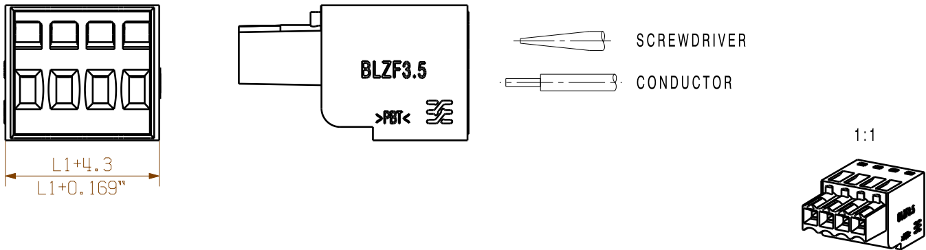
SHOWN:BLZF 3.50/04/180LR
