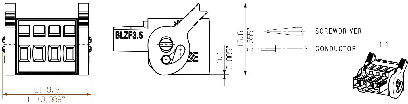
SHOWN:BLZF 3.50/04/180LH
