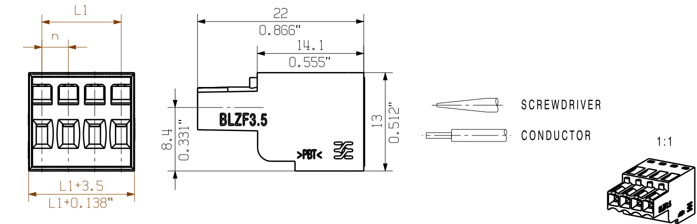
SHOWN:BLZF 3.50/04/180
