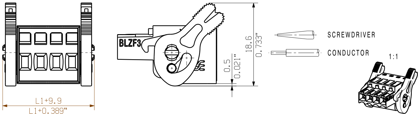
SHOWN:BLZF 3.50/04/180LR
