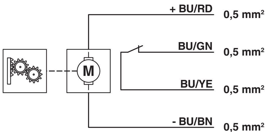
Schéma fonctionnel
