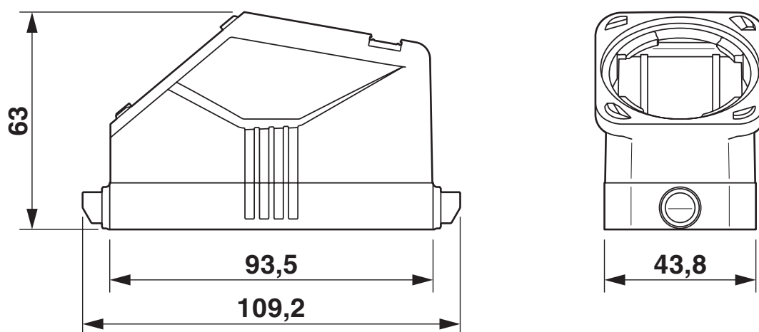
Dessin coté
