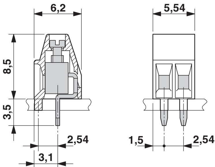
Maßzeichnung
