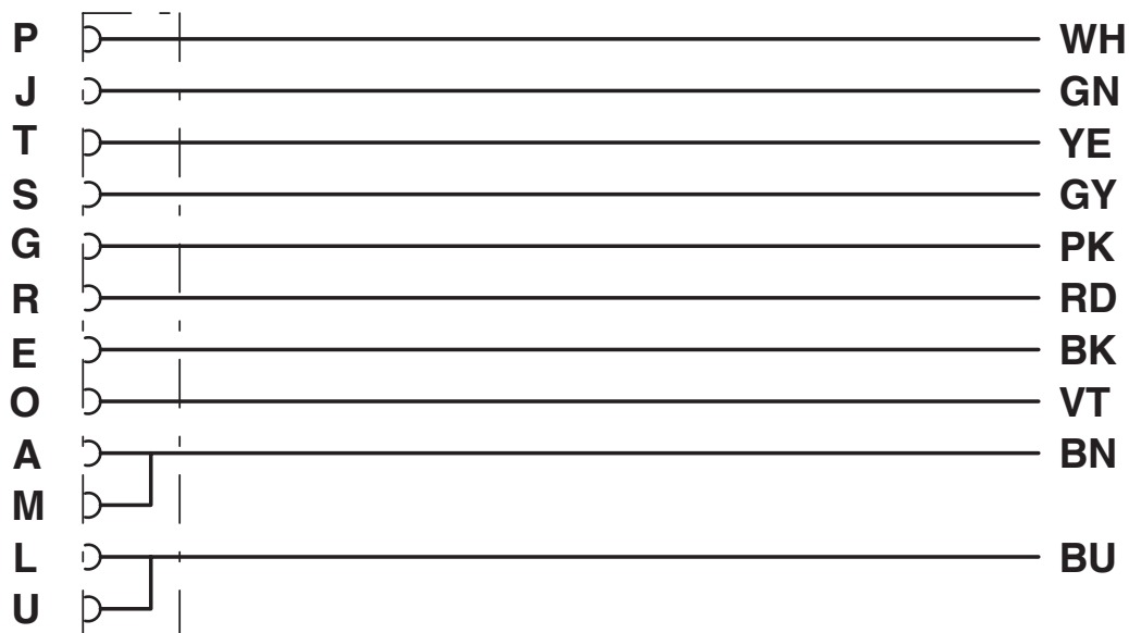
Kontaktbelegung der M16-Buchse
