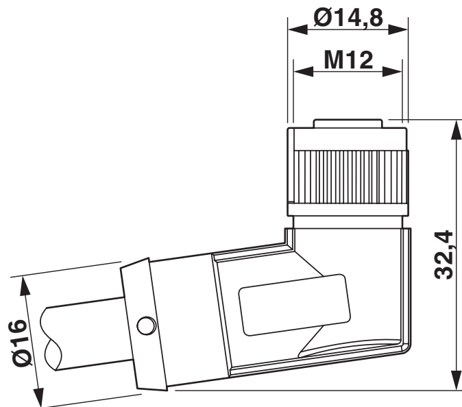
Dessin coté
