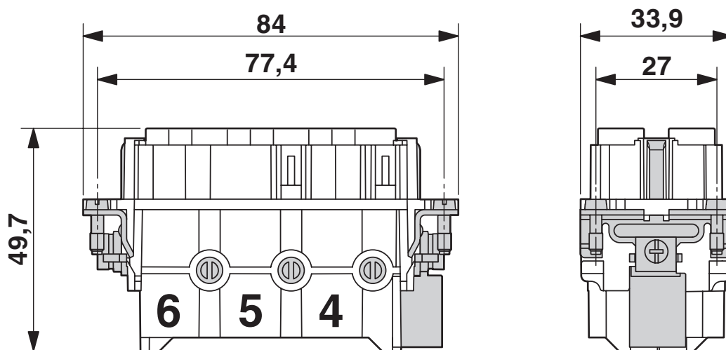
Maßzeichnung
