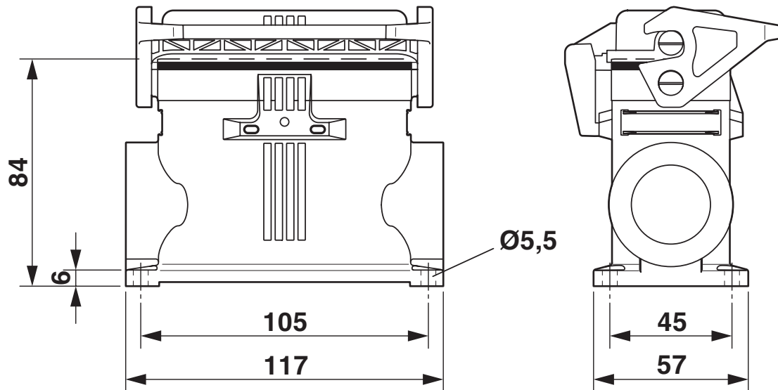
Maßzeichnung
