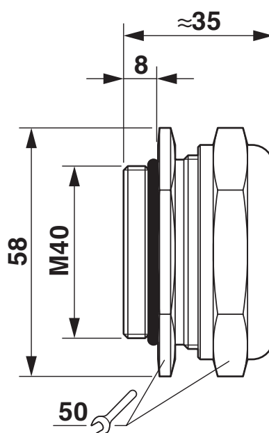
Dessin coté
