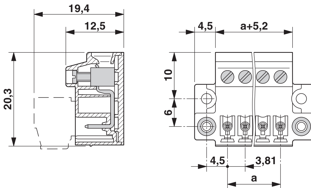
Dessin coté
