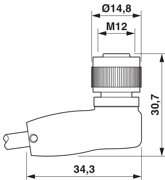
Dessin coté
