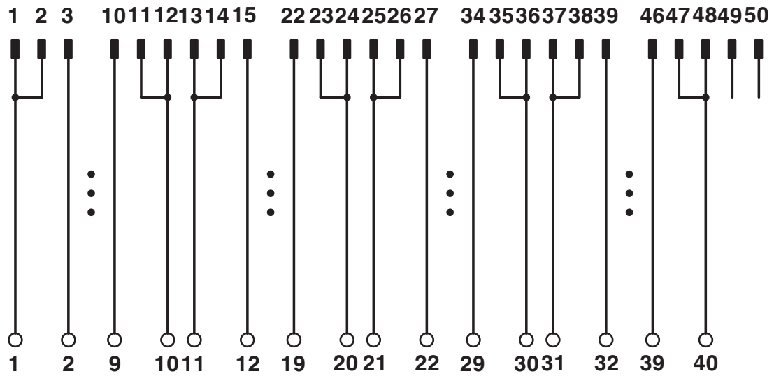
Schaltplan
