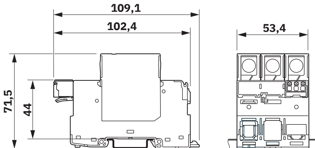
Dessin coté
