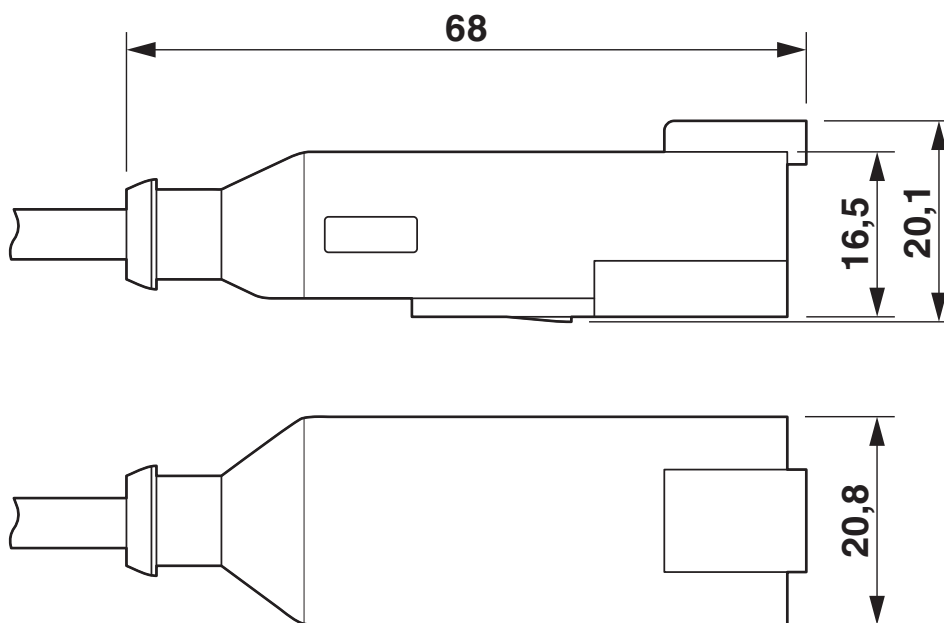
DEUTSCH DT04-4P, vista superior y lateral
