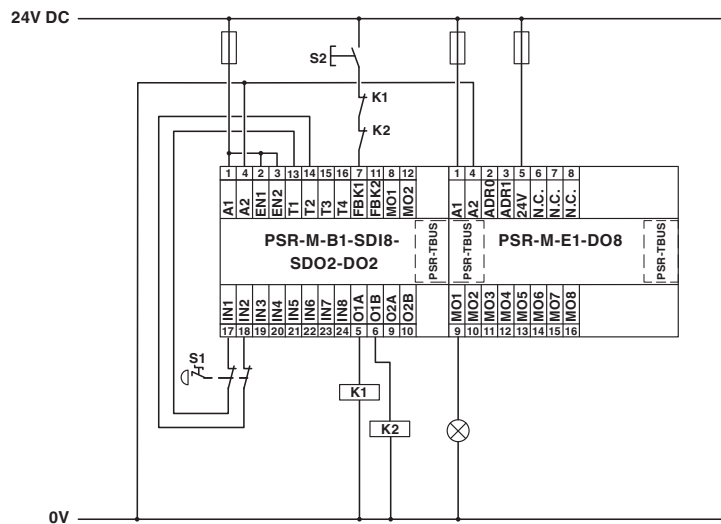
Applikationszeichnung
