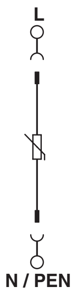
Schaltplan
