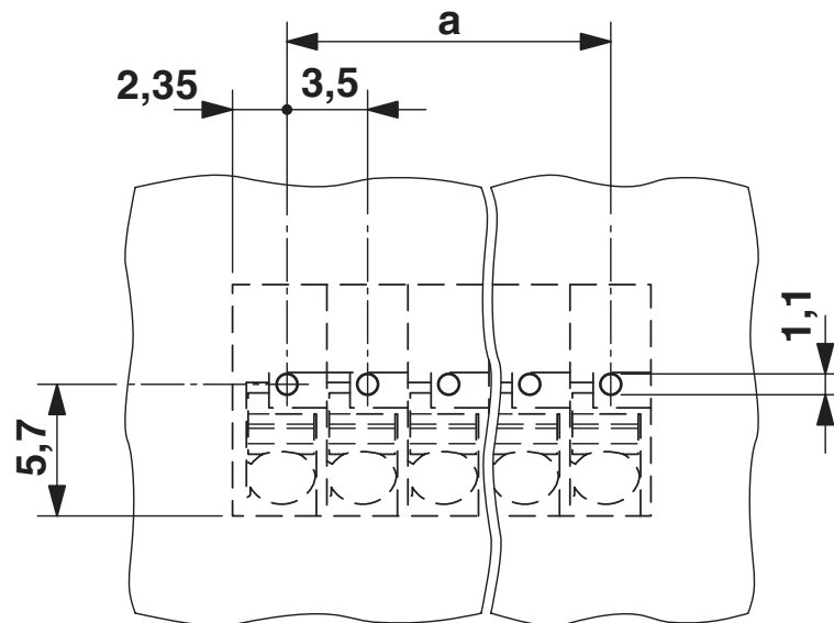
Bohrplan/Lötpadgeometrie
