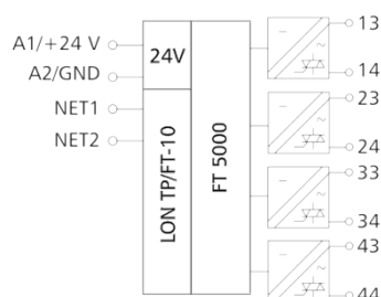
Prinzipbild
