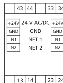
Anschlussbild
