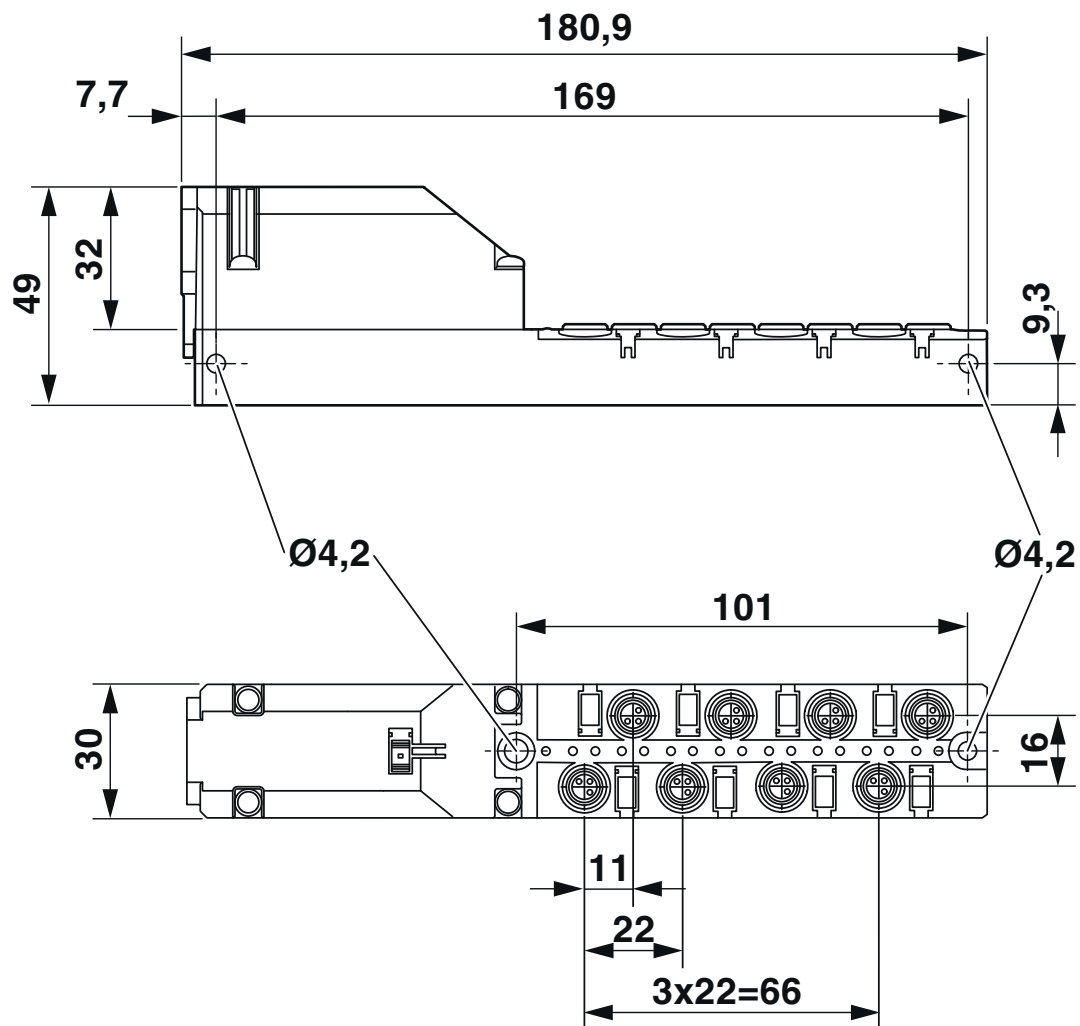
Maßzeichnung
