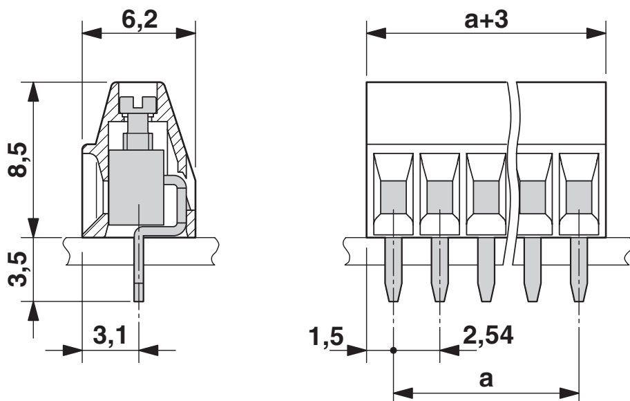
Dessin coté
