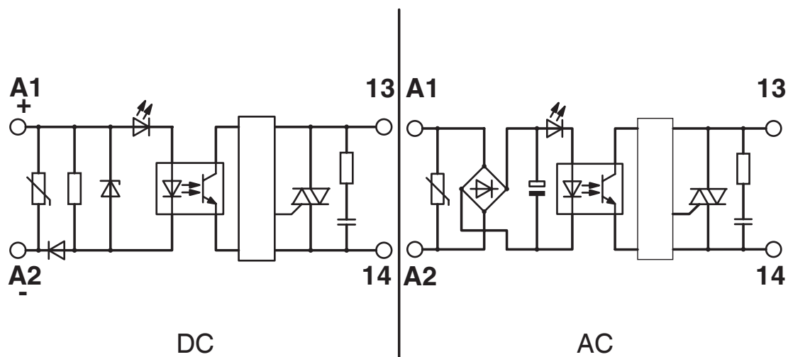
Diagrama eléctrico
