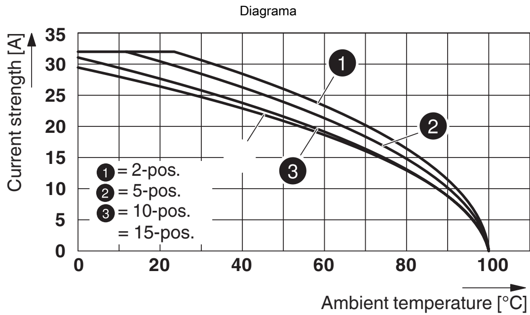
Diagrama eléctrico
