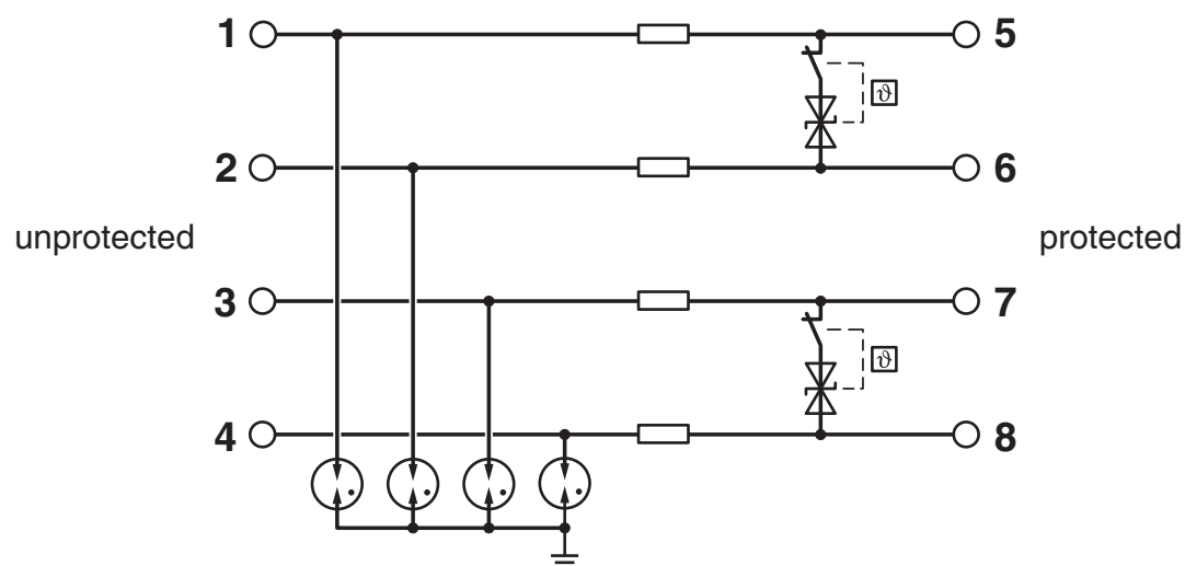
Diagrama eléctrico
