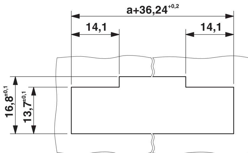
Maßzeichnung
