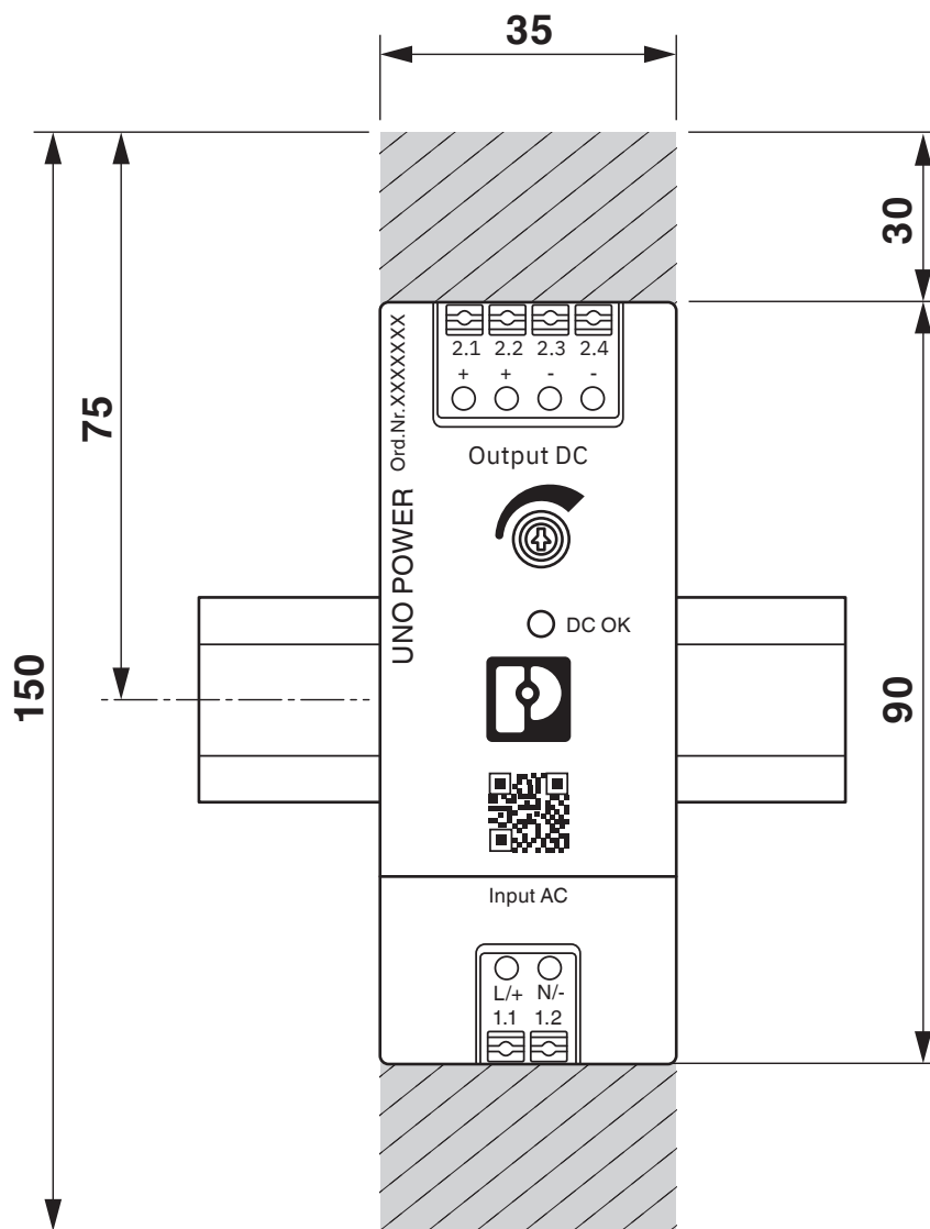
Esquema de dimensiones
