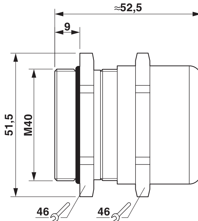
Dessin coté
