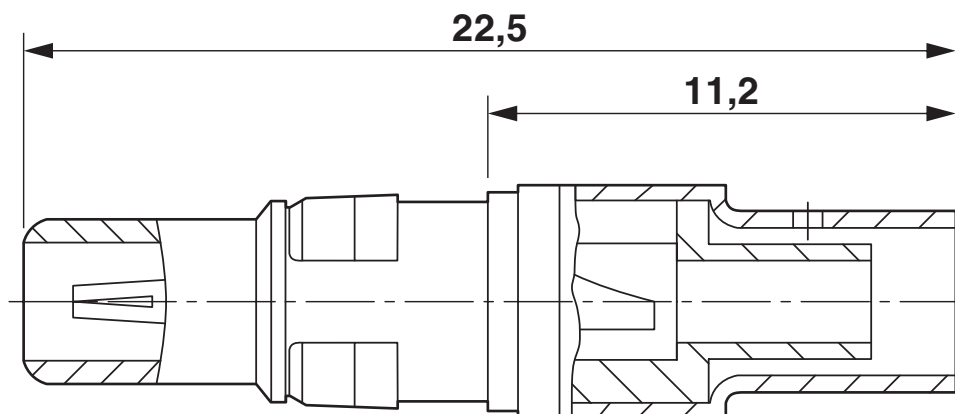
Contacto coaxial hembra D-SUB
