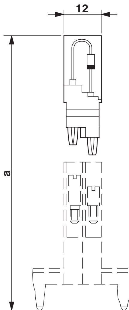
Esquema de dimensiones
