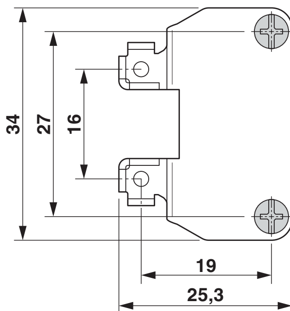
Dessin coté
